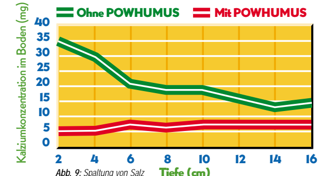
Abb. 9: Spaltung von Salz
