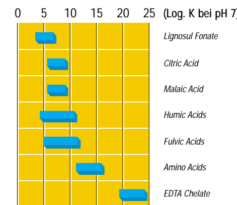
Abb. 8: Chelatstärke organischer Komplexbildner
